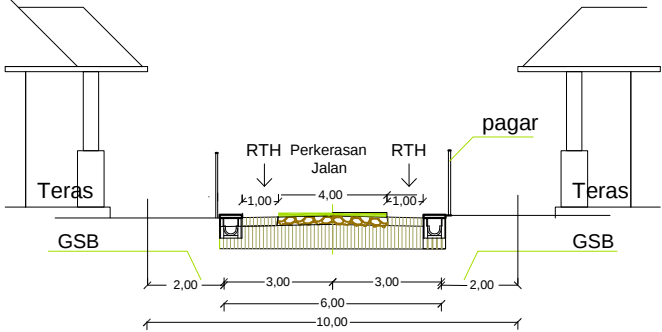
Potongan Jalan Lebar 6,00 m
